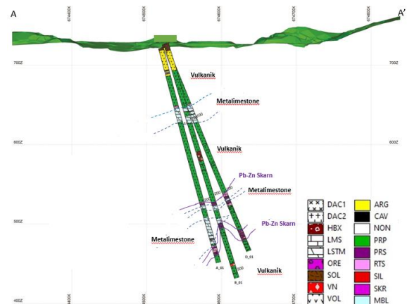
Gambar 12. Penampang lubang bor A_01, B_01, dan D_01
