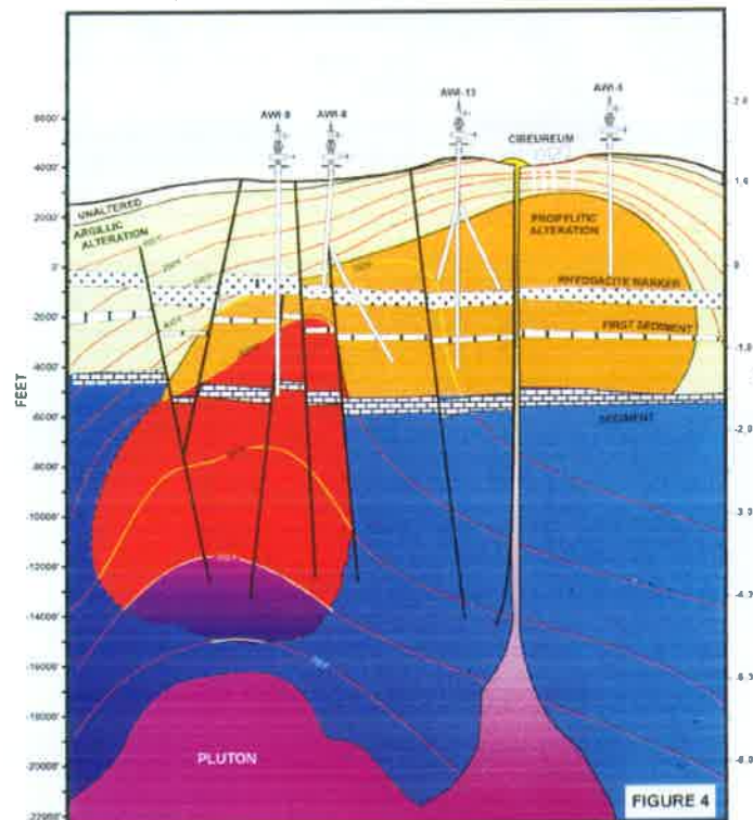
Gambar 3. Model hidrotermal Lapangan Awibengkok, Komplek Gunung Salak (CGI, 2002) (Contoh tipe sistem panas bumi kompleks vulkanik di pulau besar)
