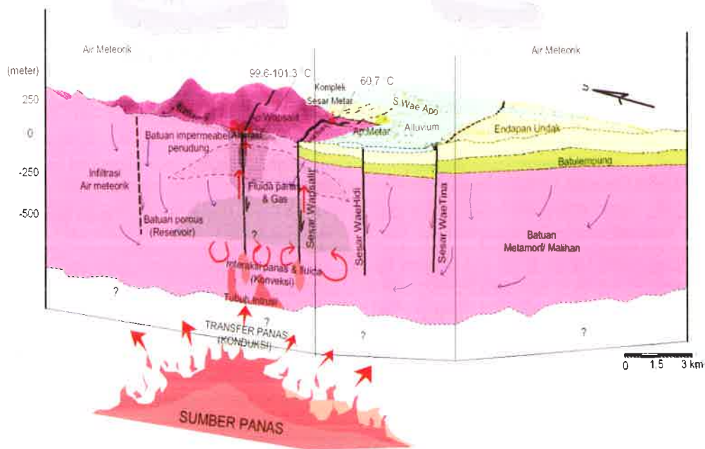
Gambar 6 : Model tentatif panas bumi Wapsalit, Buru (Badan Geologi, 2007) (Contoh tipe sistem panas bumi Non Vulkanik).
