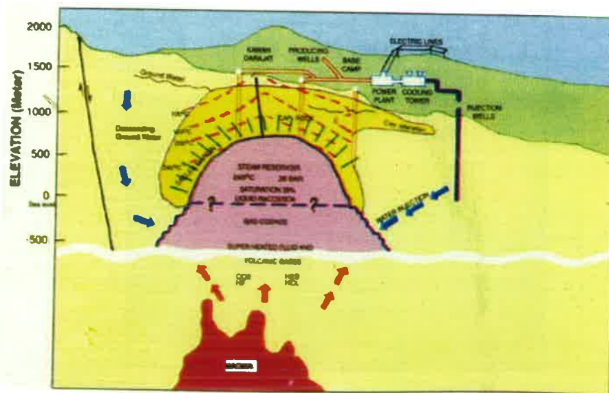
Gambar 4. Model sistem panas bumi dan fasilitas produksi Darajat, Kabupaten Garut. (CGI,1998). (Contoh tipe sistem panas bumi kaldera)
