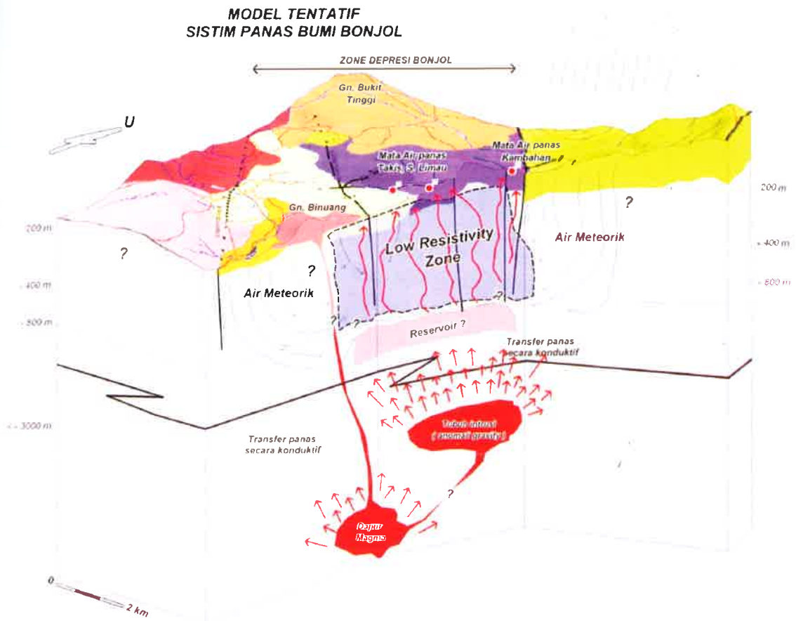
Gambar 5: Model tentatif sistem panas bumi Bonjol, Sumatera Barat (Badan Geologi, 2007) (Contoh tipe sistem panas bumi vulkano-tekonik : graben-kerucut vulkanik)
