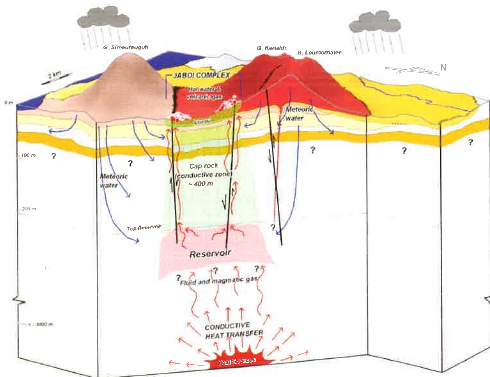
Gambar 2: Model tentatif sistem panas bumi Jaboi, Aceh (Badan Geologi, 2006) (Contoh tipe sistem panas bumi kompleks vulkanik di pulau kecil)
