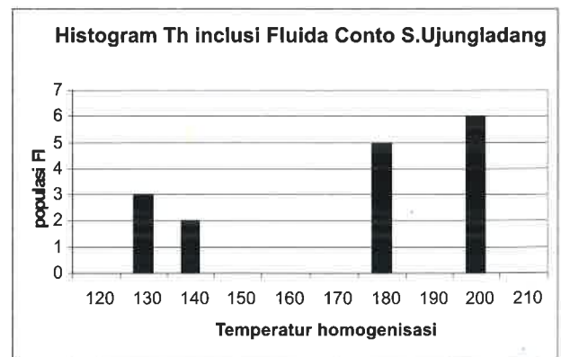
Gambar 4 Histogram Th Inklusi Fluida Contoh S
