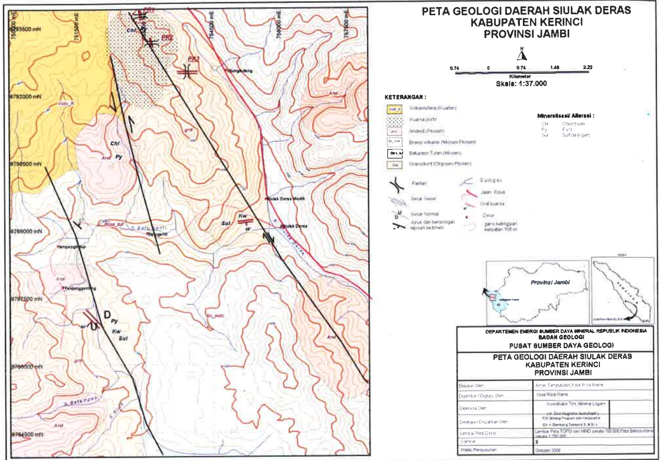
Gambar 2. Peta Geologi, Lokasi Contoh FI dan Lokasi Indikasi Endapan Logam Daerah Siulakderas Mudik dan Sekitarnya, Kabupaten Kerinci, Provinsi Jambi (Rosidi, dkk, 1996)
